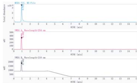
LC-MS
