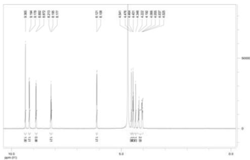
NMR
